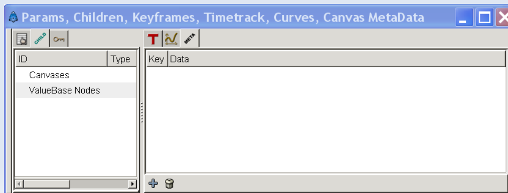
Окно панелей
