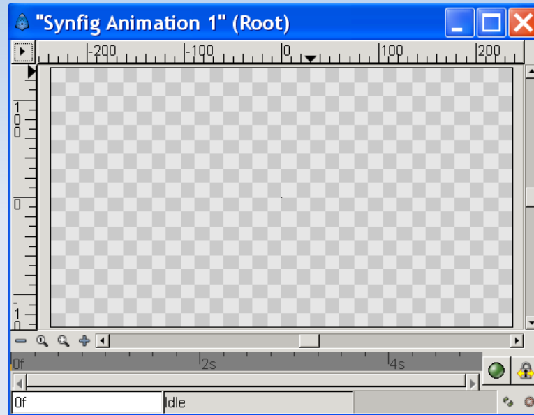
Рабочее окно
