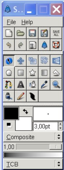
Панель инструментов
