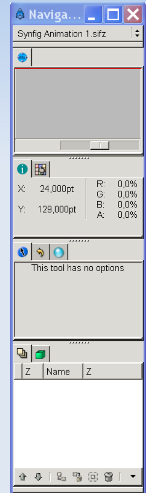
Окно панелей
